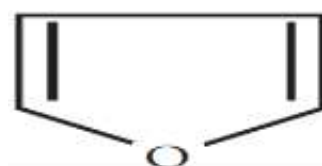
Furan VIII
