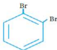
1,2 dibromobenzene
