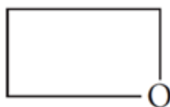
XIV oxetane
