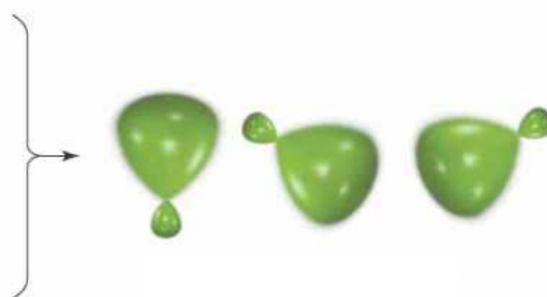
ثلاث أوربيتالات مهجنة من نوع sp^2
