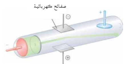
تأثر الاشعة الكاثودية بالصفائح الكهربائية.
