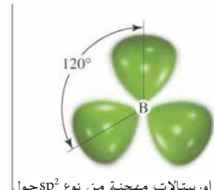
ثلاث أوربيتالات مهجنة من نوع sp^2 حول ذرة B.
