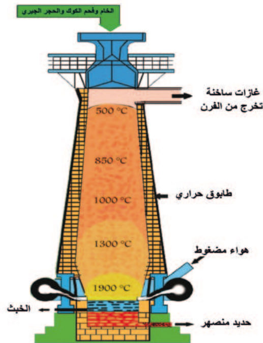
الفرن النفخ ( استخلاص الحديد )
