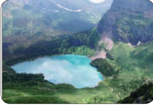
شكل (٥٨) أحد أنواع البحيرات التكتونية
