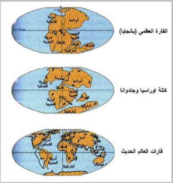
شكل (٦٧) نظرية زحزحة القارات
