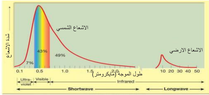
الشكل (8-1) الاشعاع الذي تشعه كل من الشمس والأرض
