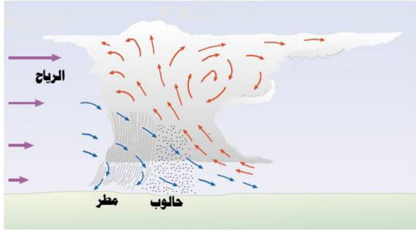
الشكل (20-1) العواصف الرعدية الشديدة
