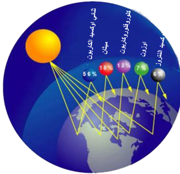
الشكل (10-1) مساهمة الغازات الدفيئة في امتصاص الأشعاع الأرضي
