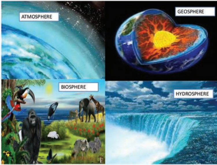
الشكل (1-1) الأنظمة الثانوية للنظام الأرضي (للاطلاع)
