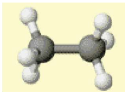
ايثان
