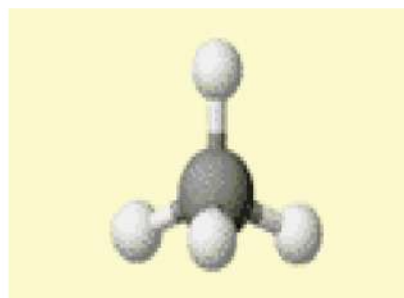
ميثان
