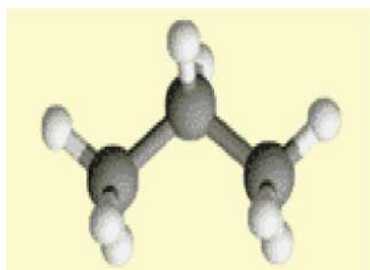
بروبان
