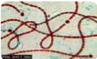
بكتيريا نوستك
